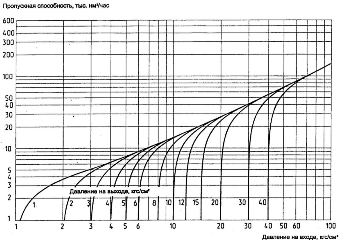
График расходных характеристик регулятора РДМ 80/200-К04
