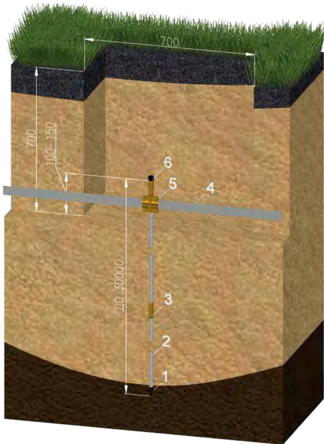
Рисунок 3. Схема монтажа УЗК на базе модульных глубинных электродов.
